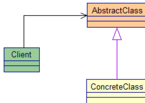
Figura 6 - L'effetto yo-yo nel pattern Template Method
