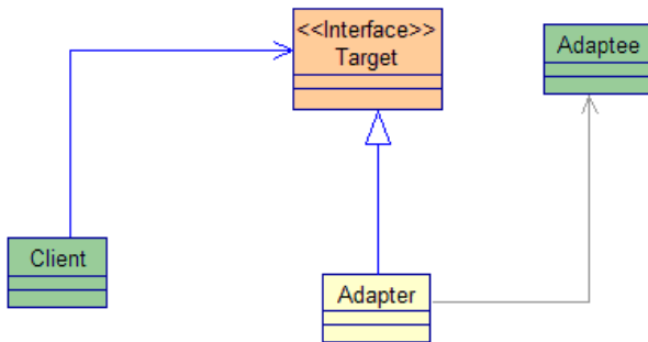
Figura 5 - La delegazione nell'Adapter
