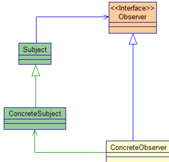
Figura 4 - La callback nel pattern Observer
