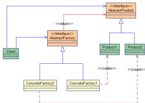
Figura 2 – Interazioni "hot potato" e chiamata fall-through nel pattern Abstract Factory
