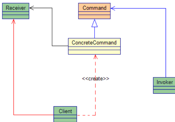
Figura 3 - Il pattern Command colorato
